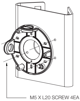
M5 X L20 SCREW 4EA
